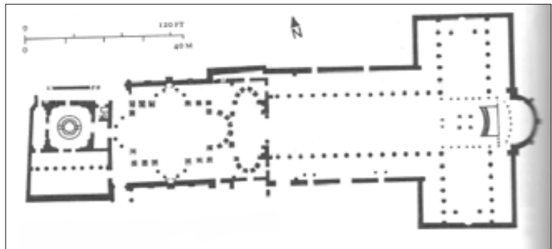
PLANTA DE L'ESGLÉSIA I EL CAPITELL, Abu Mina, Sant Menna. Construïda el 412 i reformada el 490
